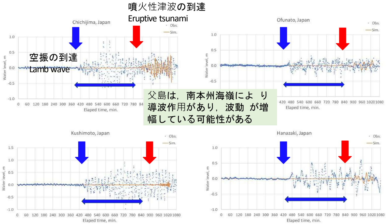
験潮記録 (青), 数值解析 (赤), 矢印は第一波の確認できる時間 (到達時間)
