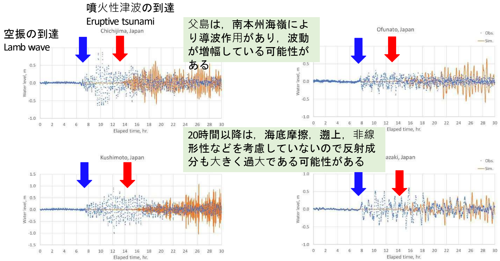
験潮記録 (青), 数値解析 (赤), 矢印は第一波の確認できる時間 (到達時間)
