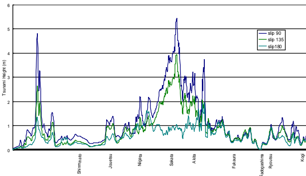
図 2 すべり方向の変化と津波高の関係
