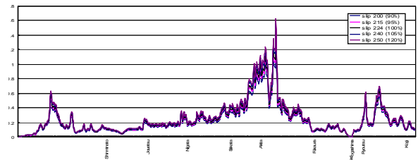
図 3 滑り量の変化と津波高の関係
